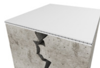
4. Vloženie tkaniny KÖSTER Flex Fabric do čerstvej prvej vrstvy
